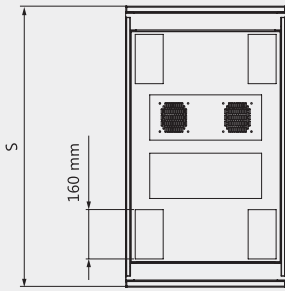
NÓC TỦ
